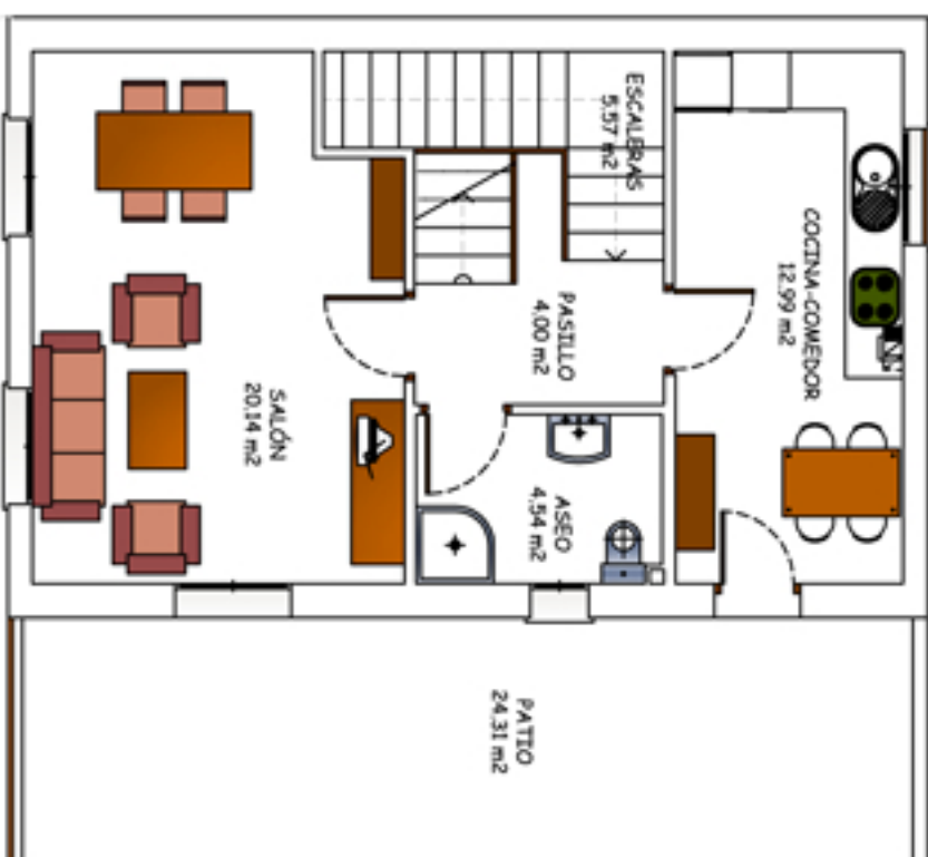
VIVIENDA TIPO 2 PLANTA PRIMERA. SUPERFICIE CONSTRUIDA: 58,90 M2
